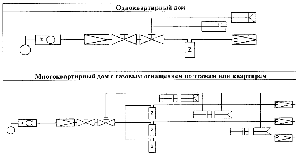
Рисунок Д.2. Активные меры безопасности при давлении в наружном газопроводе свыше 0,005 МПа до 0,6 МПа
